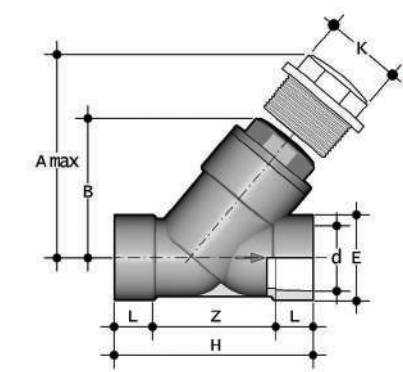
VRIV Valvola dl ritegno con attacchi femmina per incollaggio
