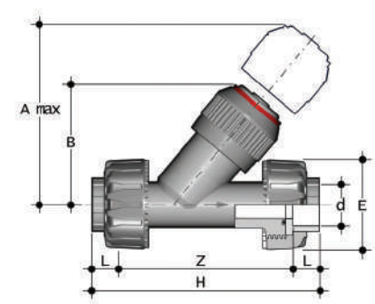
VRUIV Valvola dl ritegno con attacchi a bocchettone femmina per incollaggio
